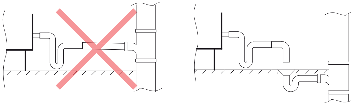
Rys. 11b. Podłączenie odpływu skroplin do kanalizacji
