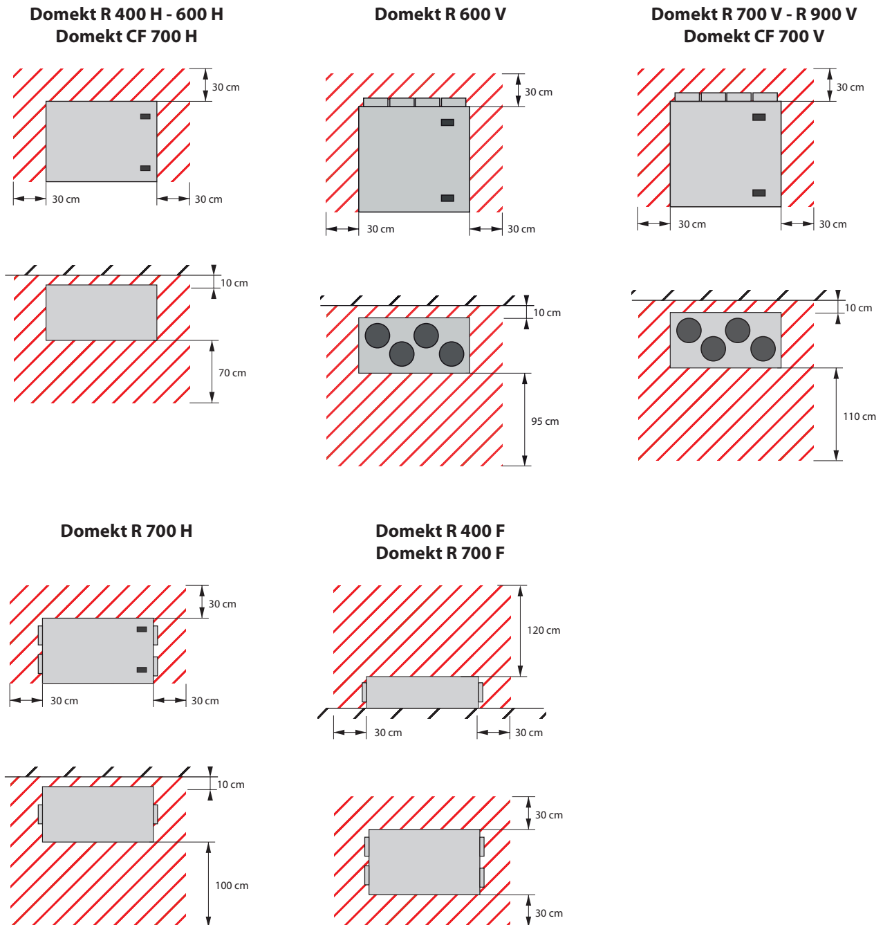
Rys. 5. Minimalna powierzchnia obsługowa
