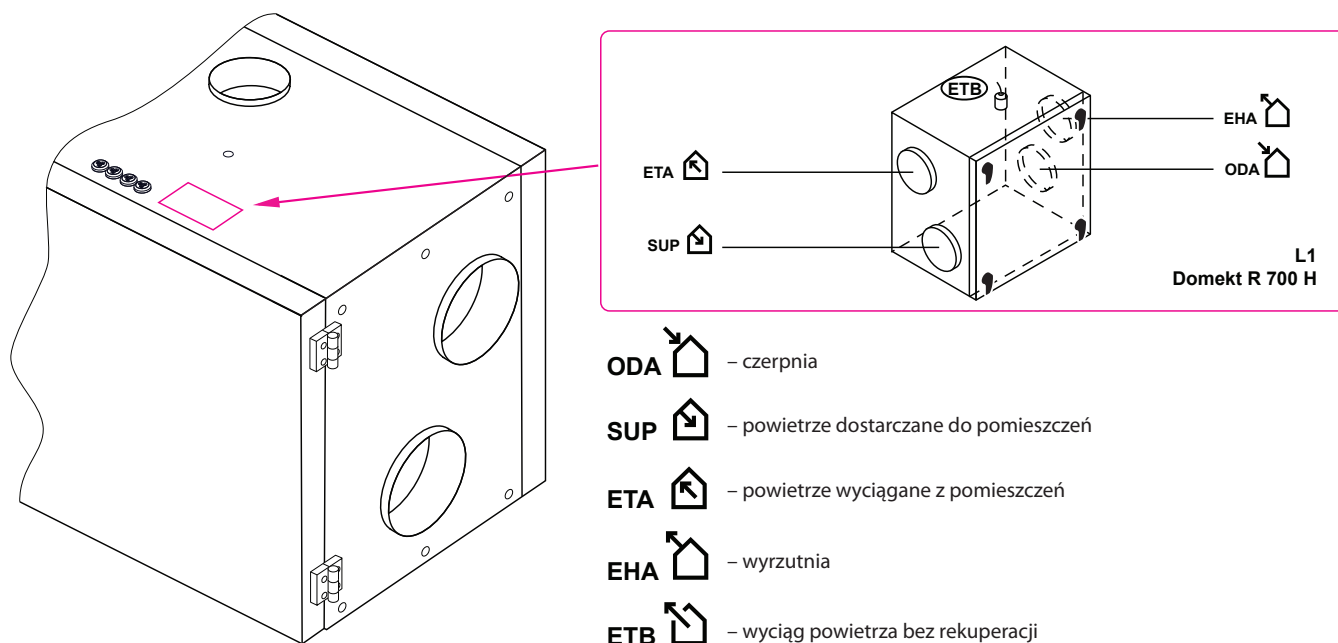
Rys. 8. Oznakowanie kanałów powietrznych
