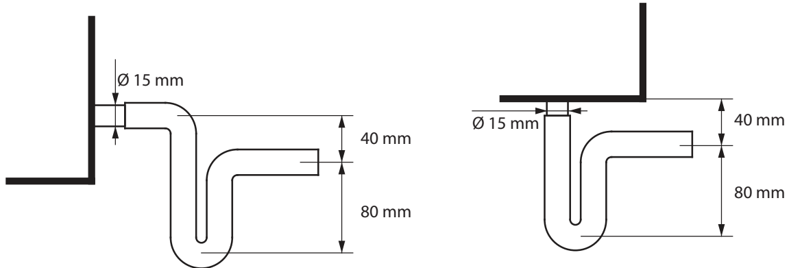
Rys. 11a. Montaż syfonu bez zaworu kulowego
