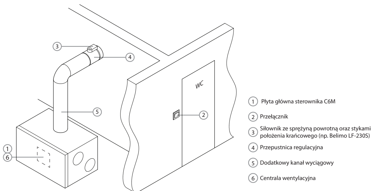
Rys. 9. Przykład montażu dodatkowego kanału wyciągowego
