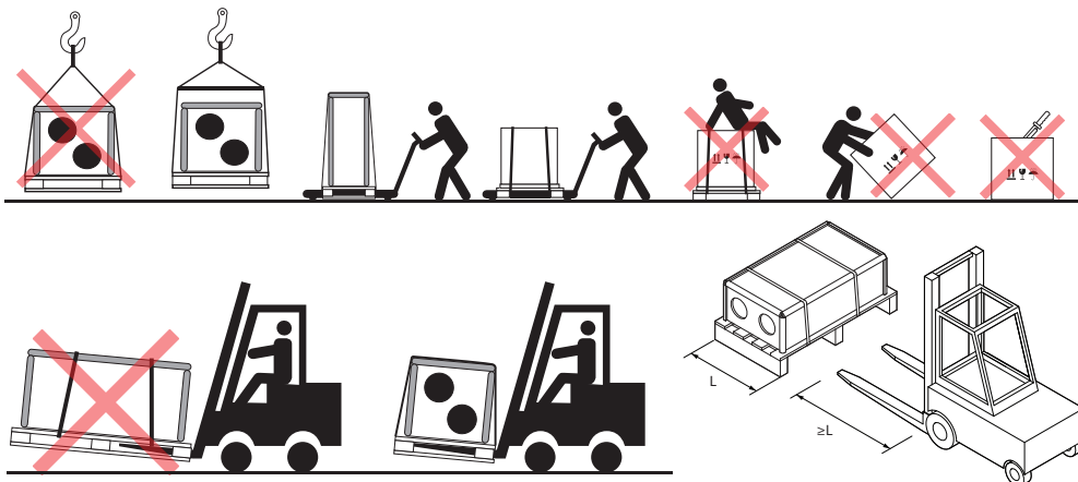
Rys. 4. Przykłady transportu dźwigiem, wózkiem widłowym lub paletowym.
